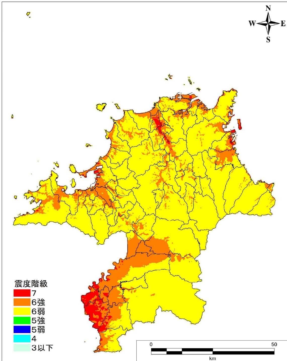
震度分布図
