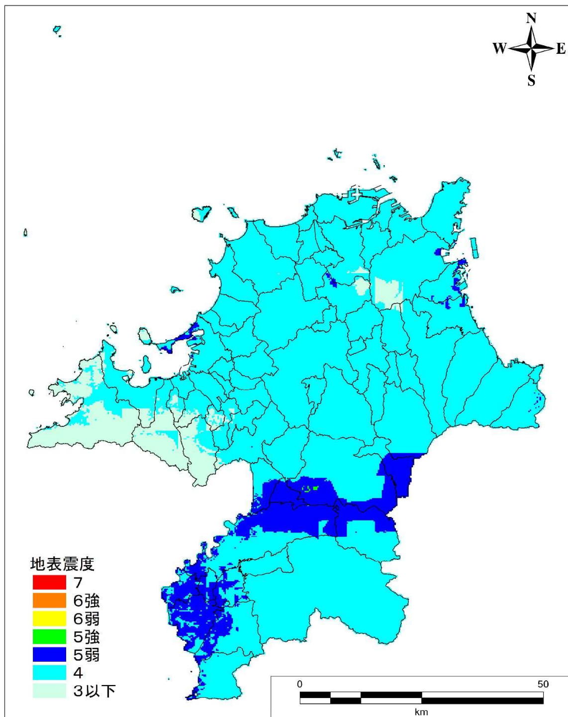
地表震度分布図 【南海トラフ（陸側ケース）】
