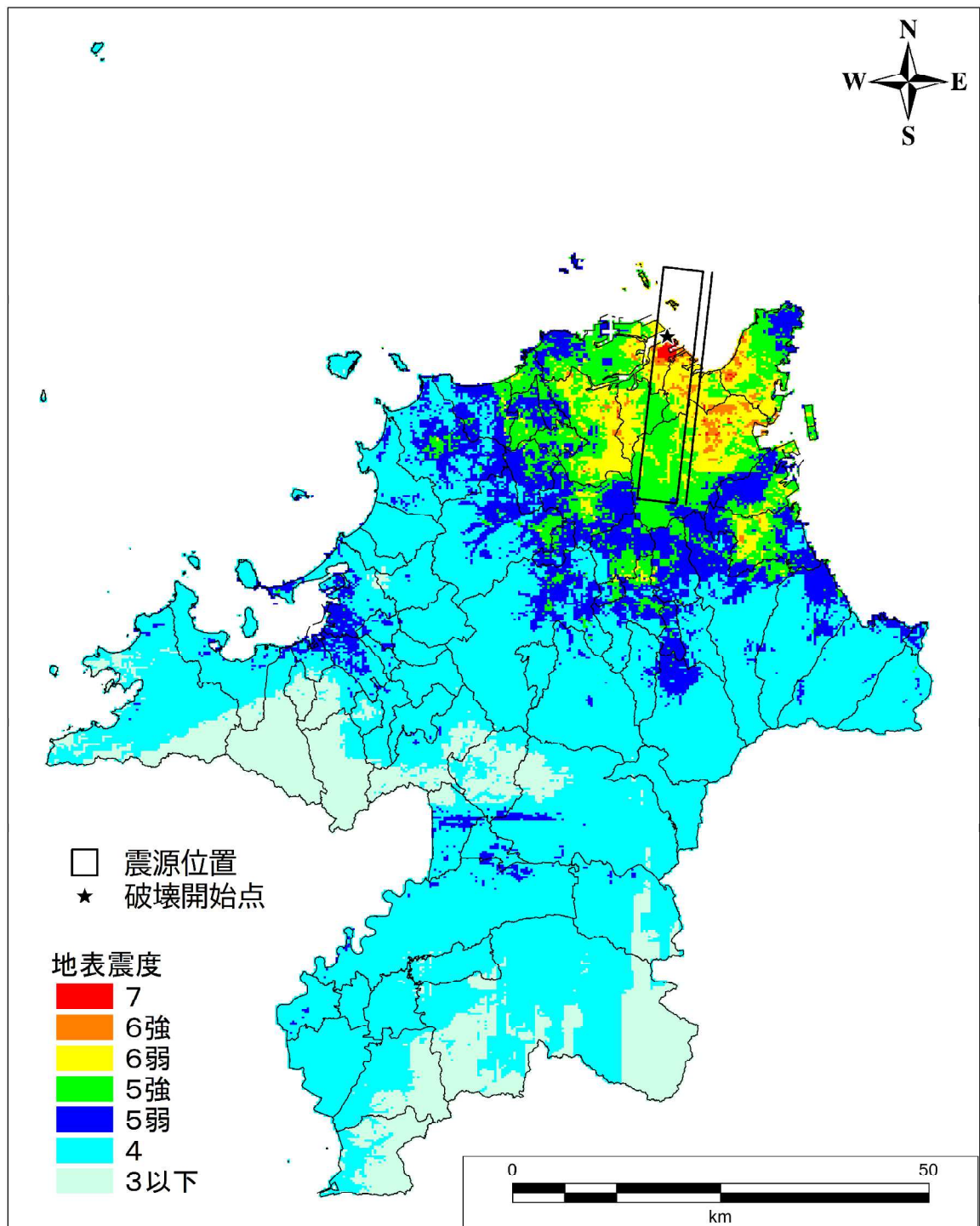
地表震度分布図 【小倉東断層（破壊開始点：北側）】
