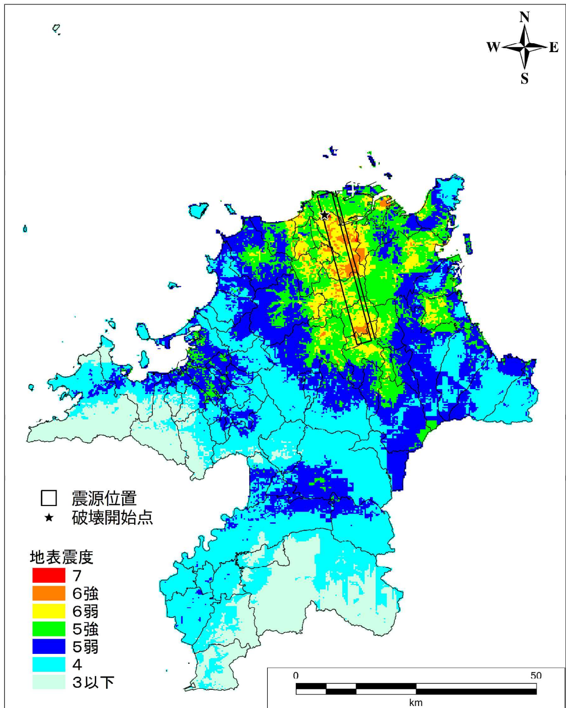
地表震度分布図 【福智山断層帯（破壊開始点：北側）】
