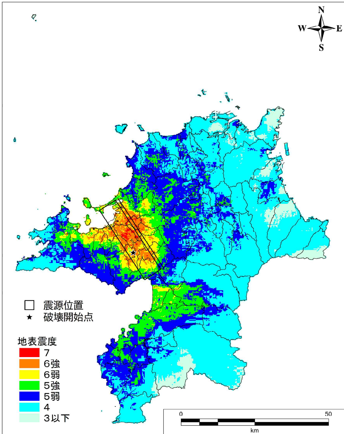
地表震度分布図 【宇美断層（破壊開始点：南側）】
