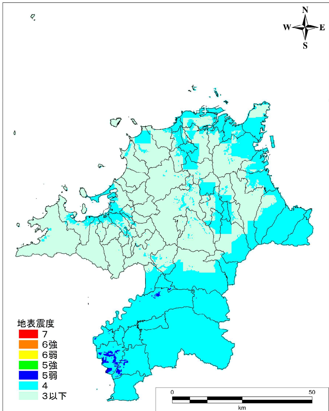
地表震度分布図 【南海トラフ（基本ケース）】
