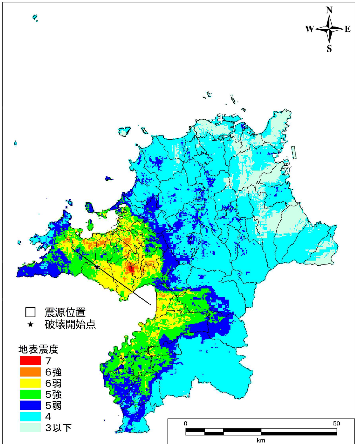
地表震度分布図
