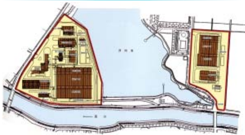
処理場平面図
