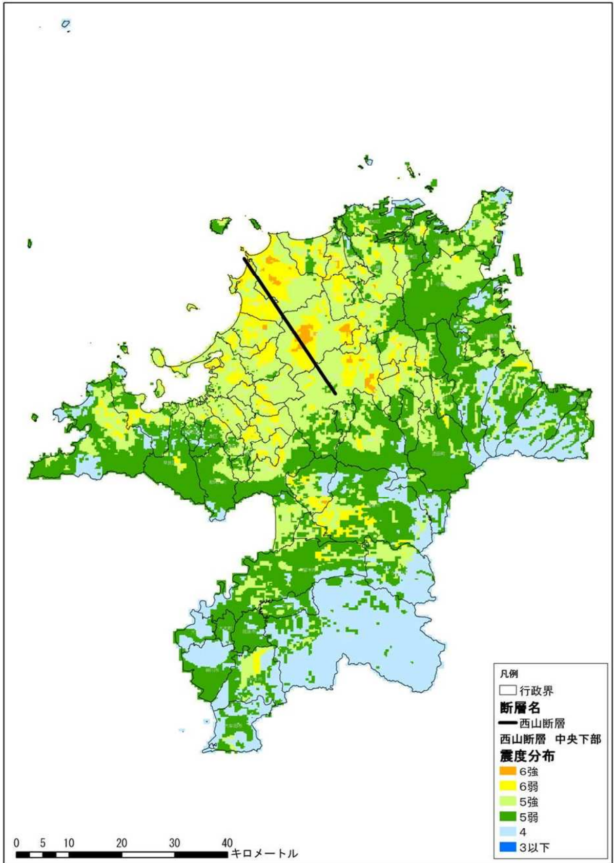
(3) 震度分布図【西山断層（破壊開始：中央下部）】
