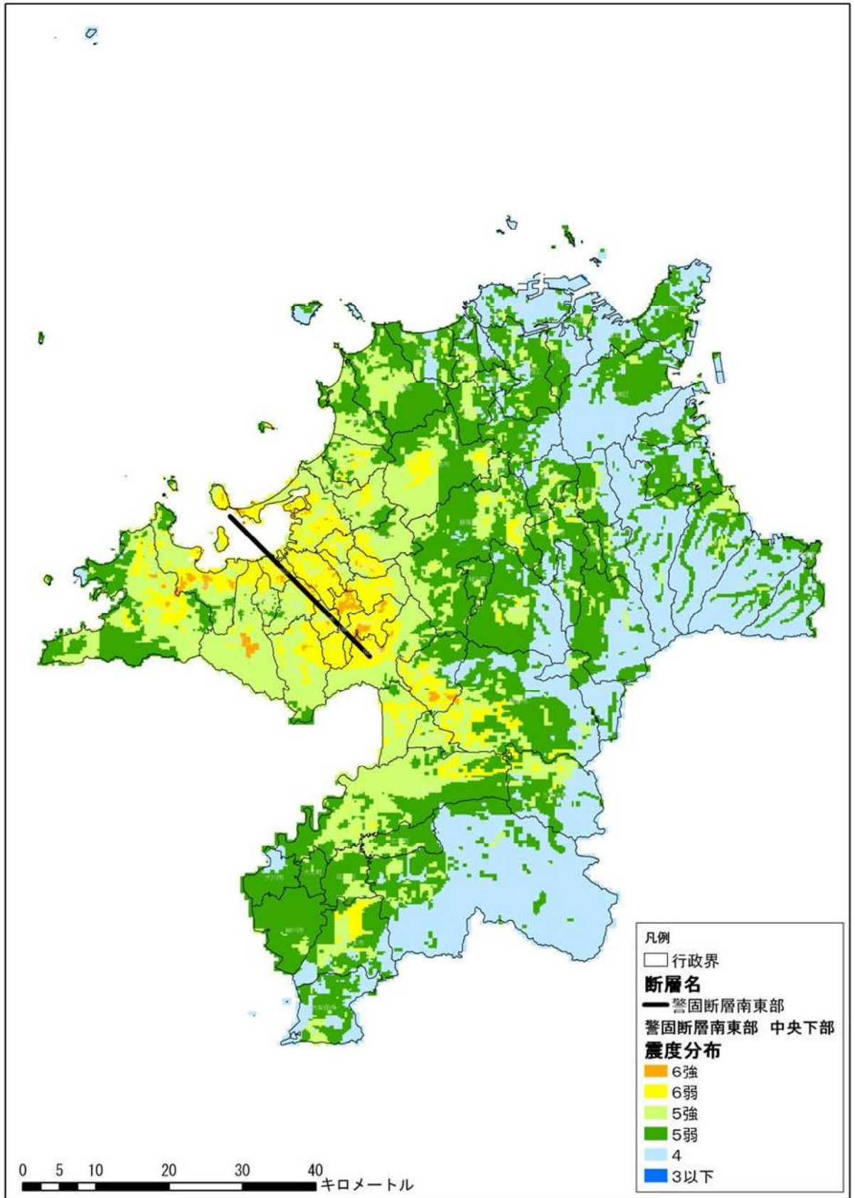
(6) 震度分布図【警固断層（南東部）（破壊開始：中央下部）】
