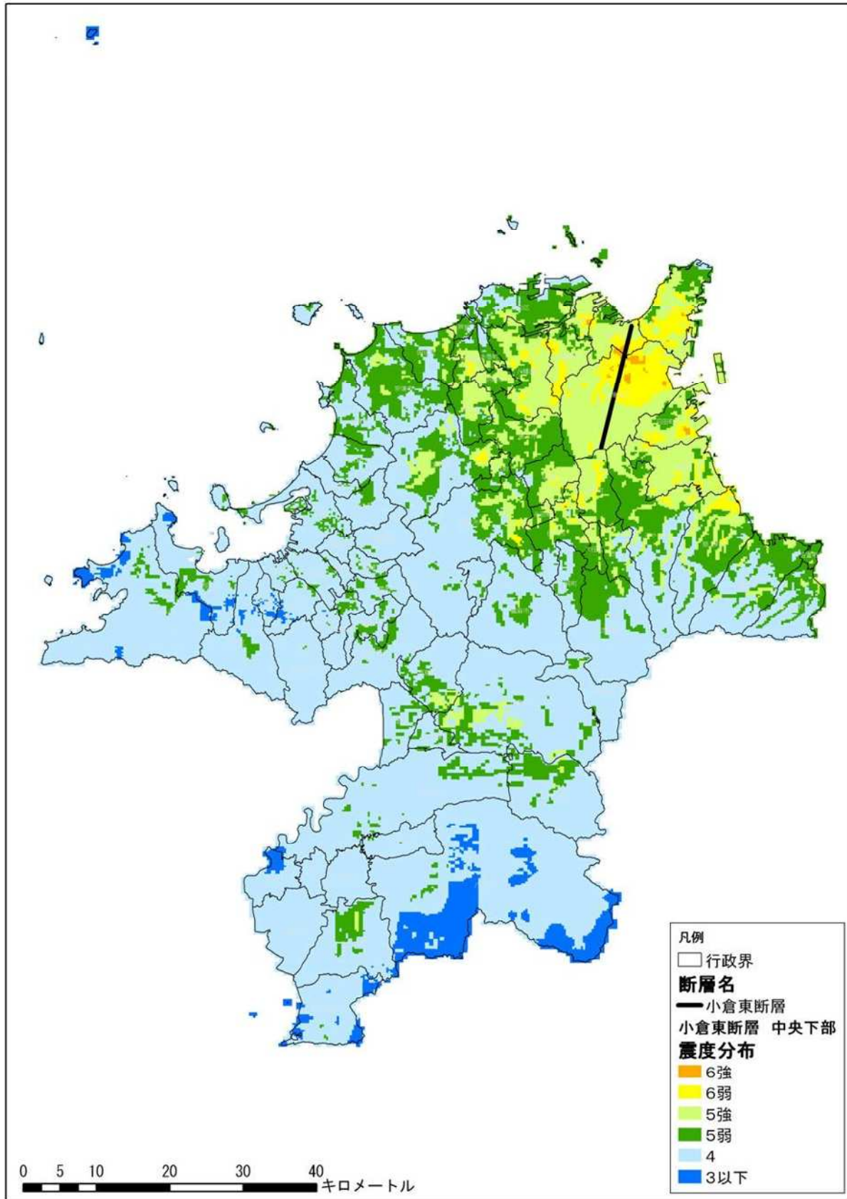
(1) 震度分布図【小倉東断層（破壊開始：中央下部）】
