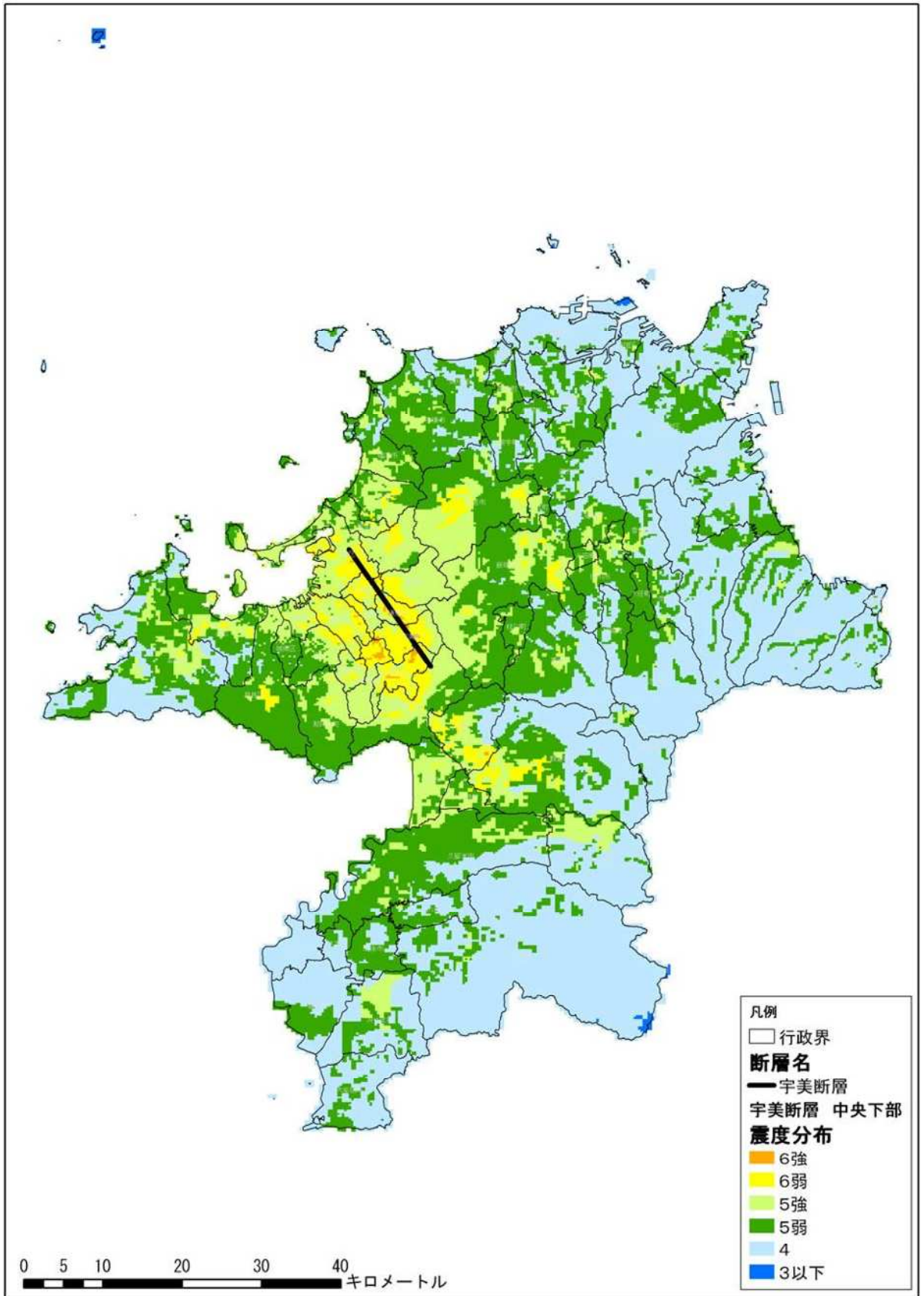
(8) 震度分布図【宇美断層 (破壊開始：中央下部)】
