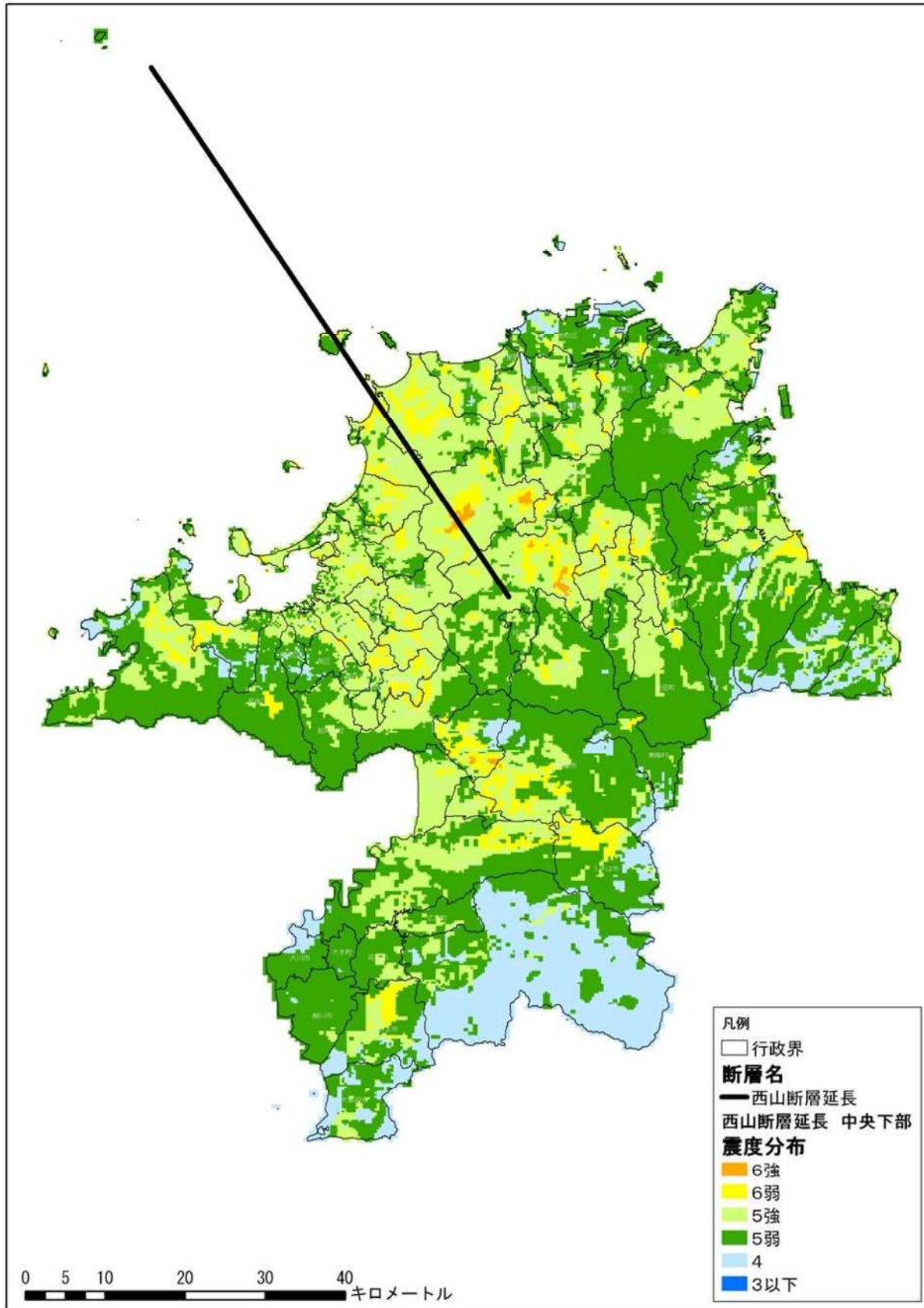
(4) 震度分布図【西山断層（延長）（破壊開始：中央下部）】
