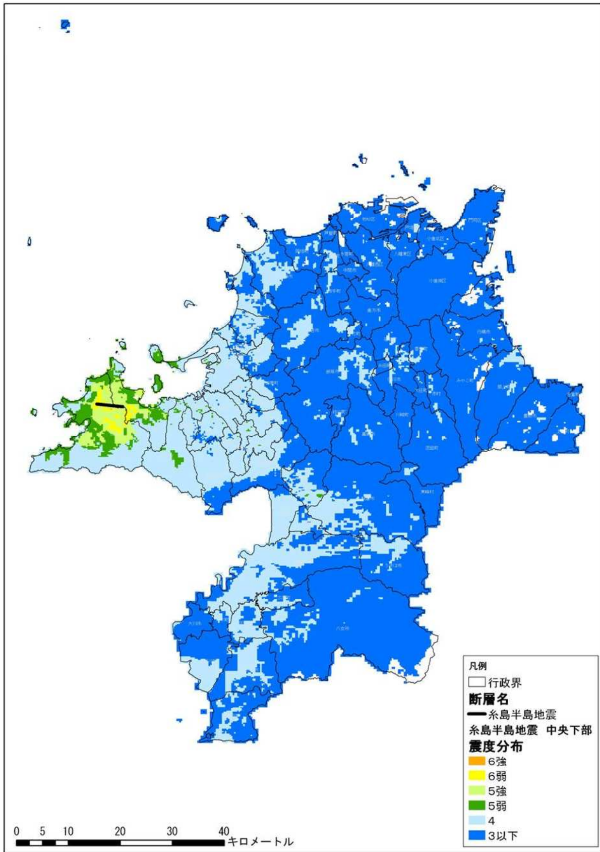
(9) 震度分布図【糸島半島の地震（破壊開始：中央下部）】
