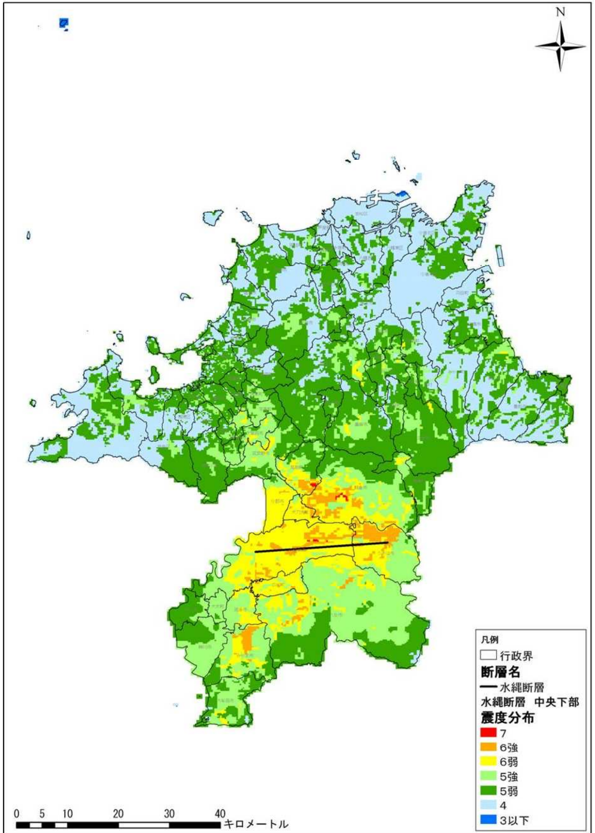
(7) 震度分布図【水縄断層（破壊開始：中央下部）】
