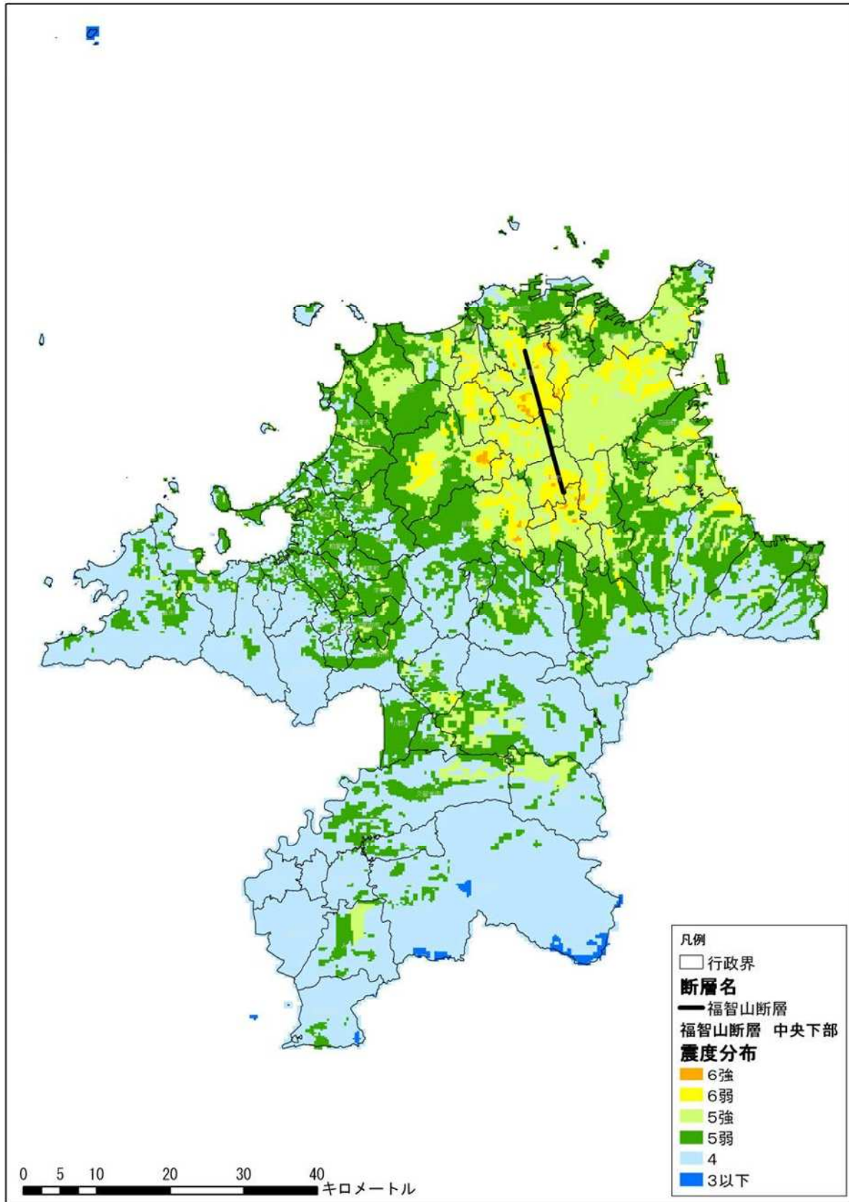
(2) 震度分布図【福智山断層(破壊開始:中央下部)】
