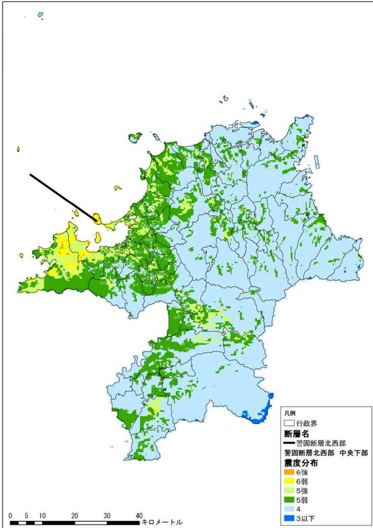
(5) 震度分布図【警固断層（北西部）（破壊開始：中央下部）】
